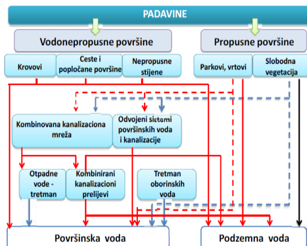
Slika 7. Održivo upravljanje oborinskim tokovima i u urbano okruženje grada Prijedora
